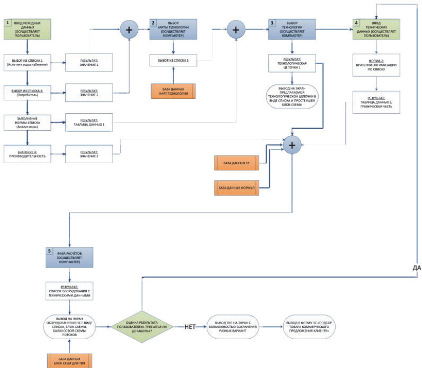
Рисунок 1. Общий алгоритм действий информационной системы IMSSE.
