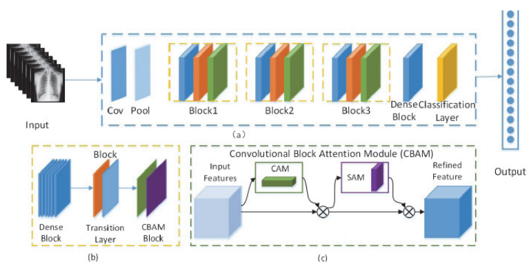
Рисунок 2. Структура модели AM_DenseNet Model [20].
