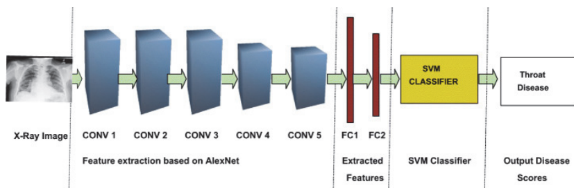
Рисунок 1. Метод SVM-AlexNet [19].
