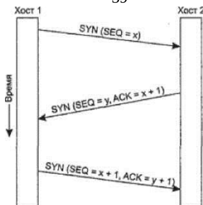
Рисунок 2 - Тройное рукопожатие
