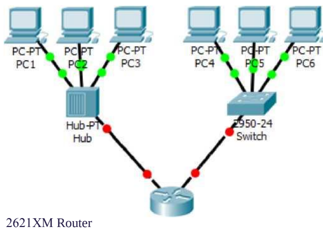
Рисунок 5 - Модель сети
