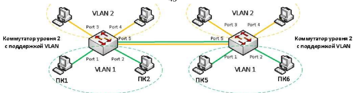
Рисунок 2 - Распределенная VLAN-сеть
