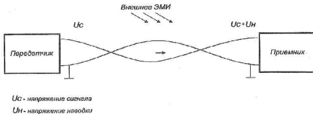
Рисунок 4 - Несимметричная сеть
