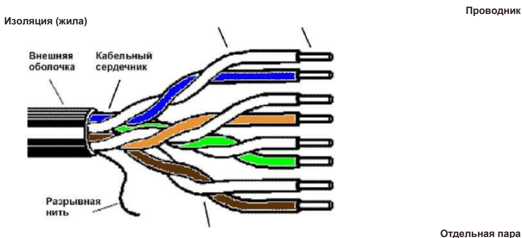
Рисунок 1 - Витая пара (8 проводников, 4 пары) (100Base-T4)
