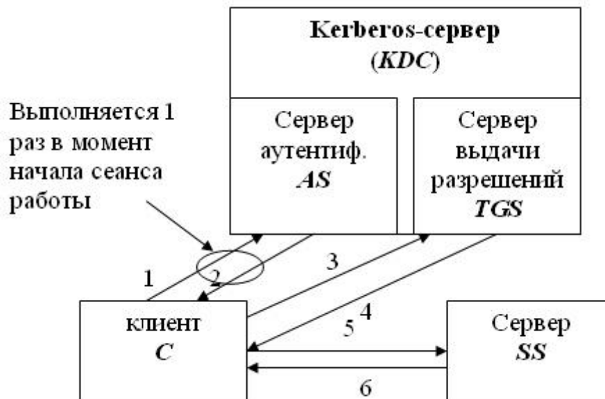
Рис. 9. Протокол Kerberos
