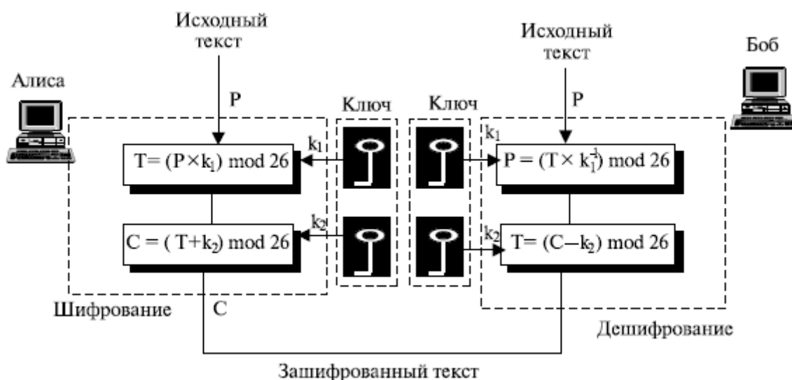
Рис. 4. Аффинный шифр
