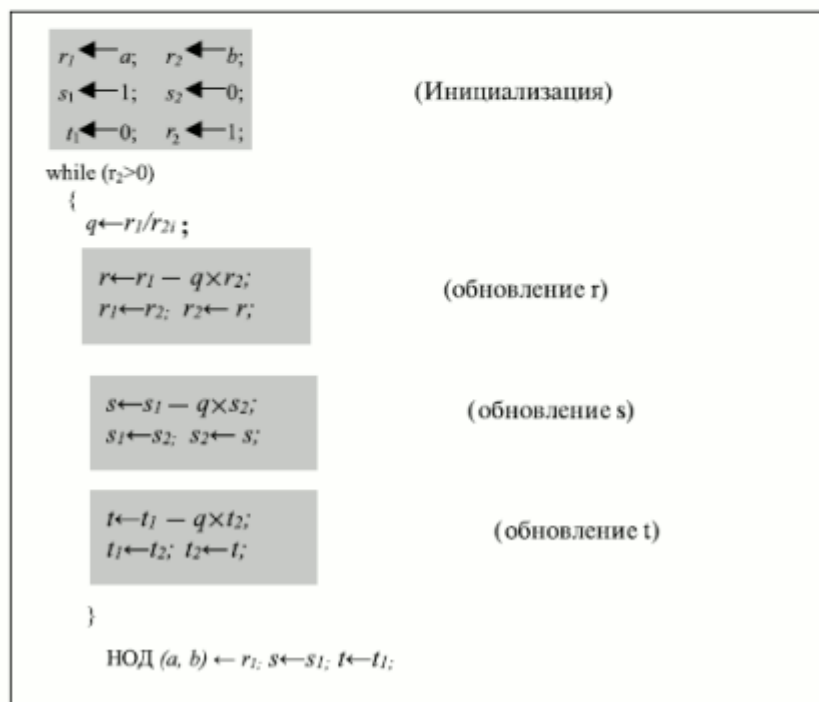
б) Алгоритм
