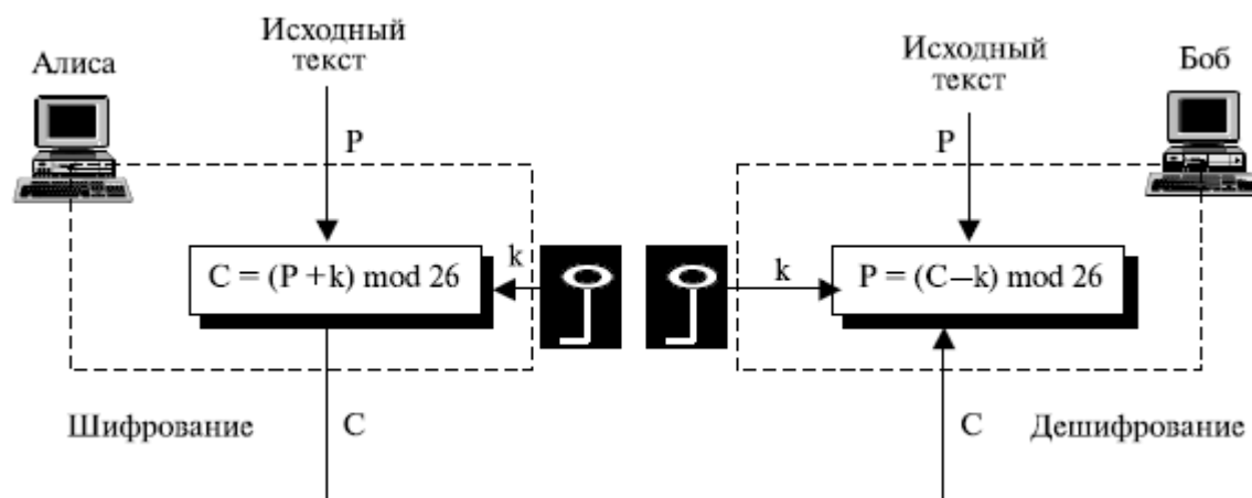
Рис. 3. Аддитивный шифр
