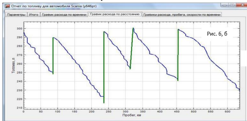
Рис. 5б. Расход топлива (л) в зависимости от пробега (км) спустя полгода после установки датчиков расхода топлива
