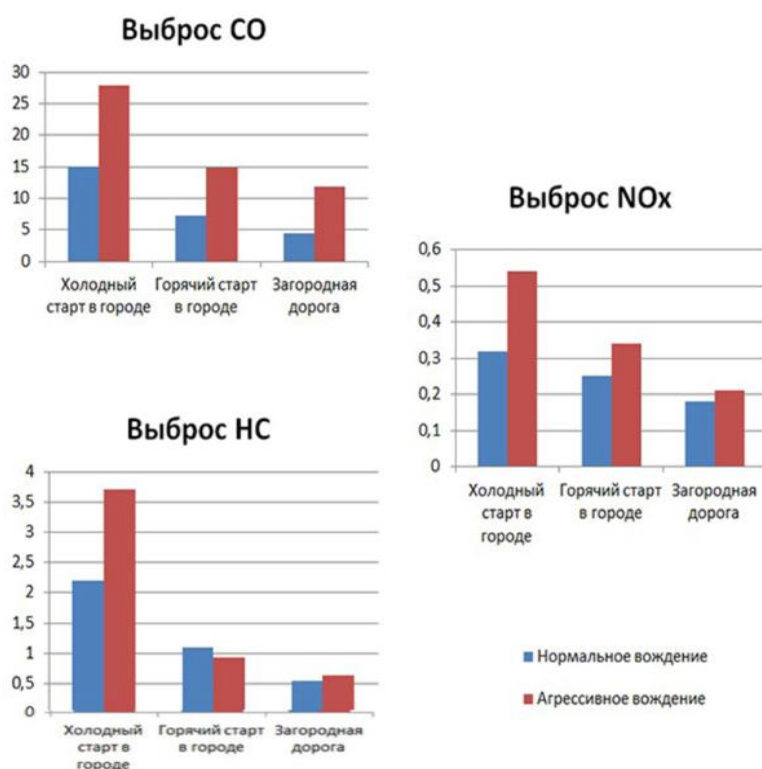
Рис. 3. Влияние выбросов вредных веществ в зависимости от режима движения.
