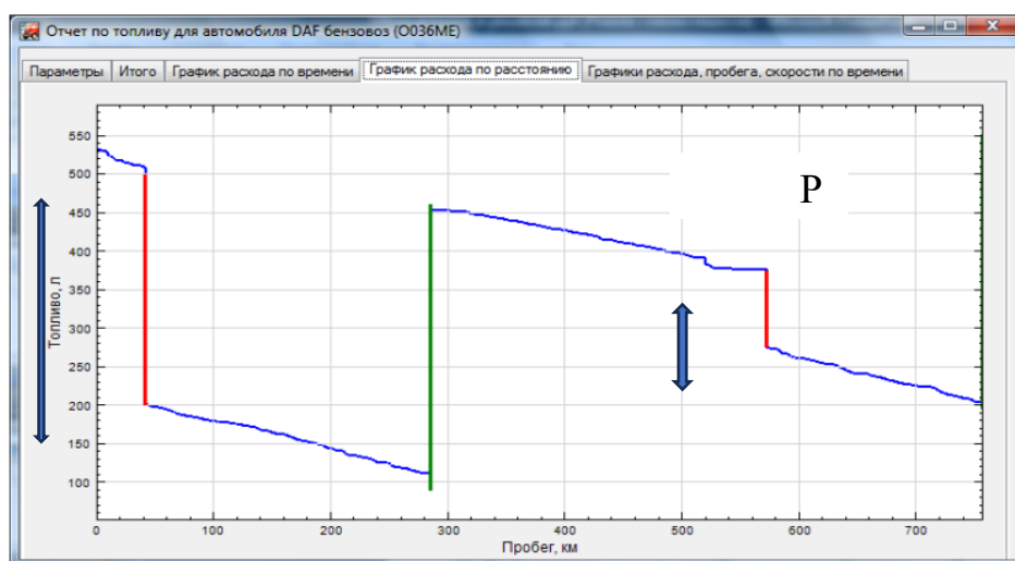
Рис. 5а. Расход топлива (л) в зависимости от пробега (км) сразу после установки датчиков расхода топлива.
