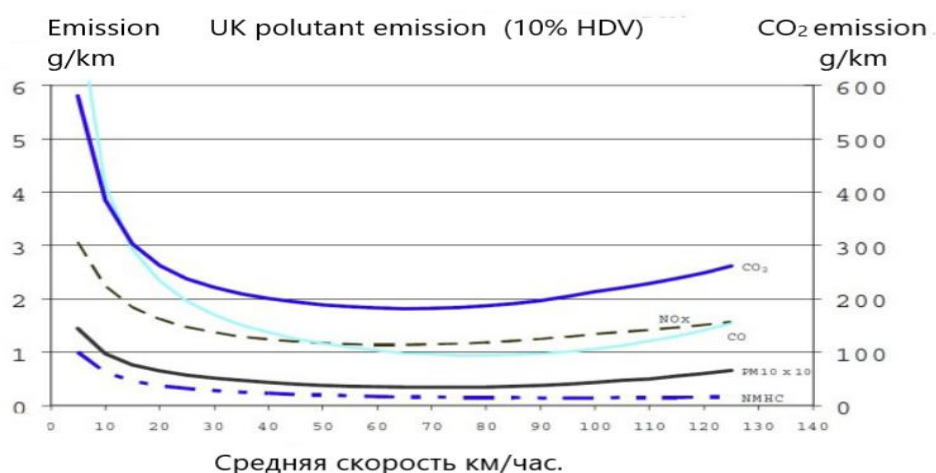
Рис. 2. Количество выброса вредных веществ в зависимости от скорости автомобиля.
